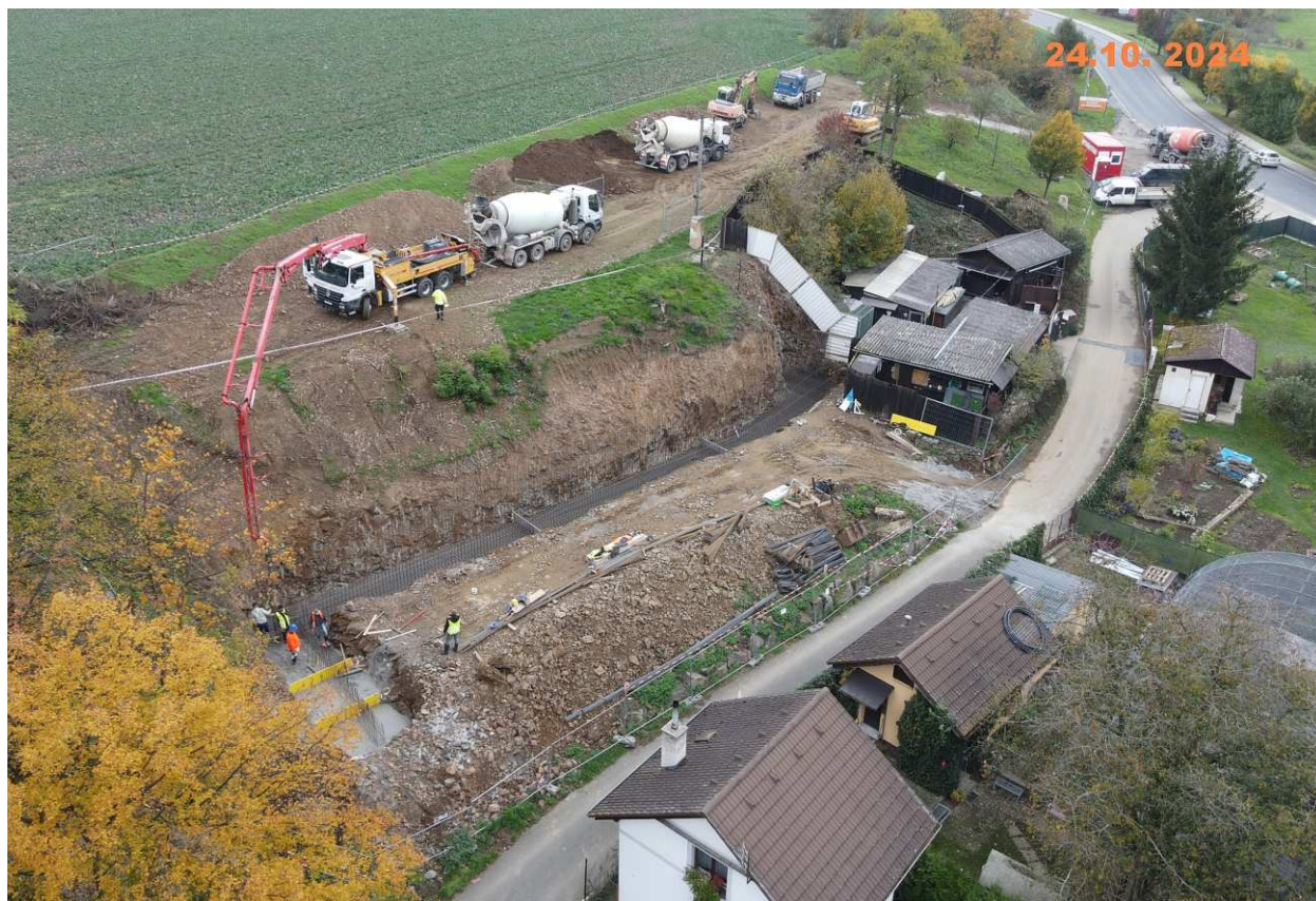
Lití betonového základu první opěrné stěny SO12.
